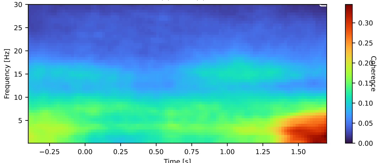
8B (4) - dPFC (6)
